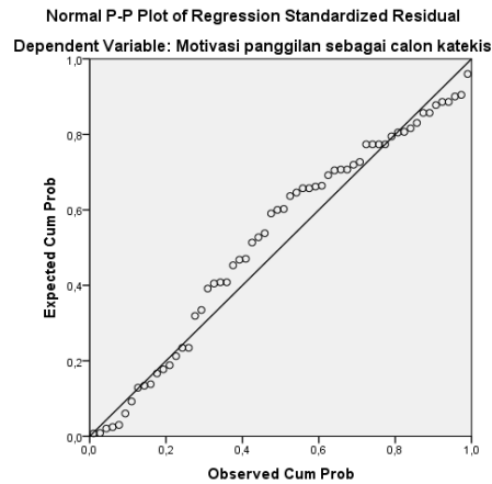
Gambar. 4.3. Normal P-P Plot Regresi
